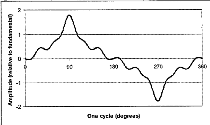
Figura 2 Amplitud de corriente para onda pico
