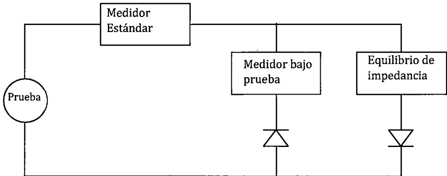
Figura 4 Circuito propuesto para prueba de corriente DC y armónicos pares (solo se muestran los circuitos de corriente de una fase, la tensión se conecta normalmente)
