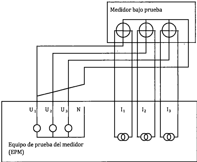
Figura 5 Montaje para la prueba de falla a tierra
