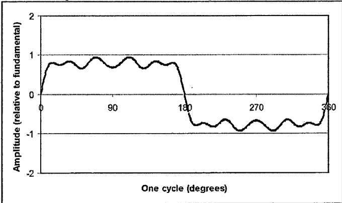
Figura 1 Amplitud de corriente para onda cuadriforme
